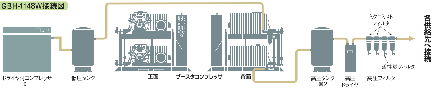
GBHV複数台接続図
