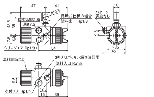
A110L 操作回路はp.10のB
