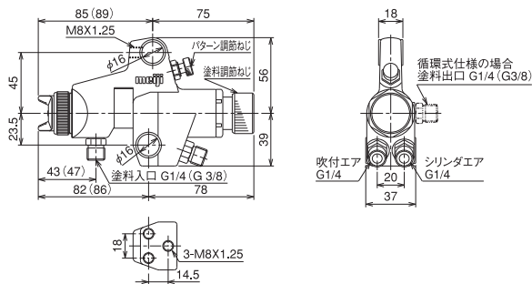
FA110・FA210・FA110L 操作回路はp.10のA
