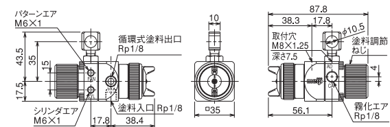
AD 操作回路はp.10のD
