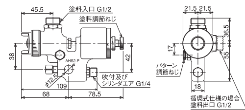
AHS2A 操作回路はp.10のC
