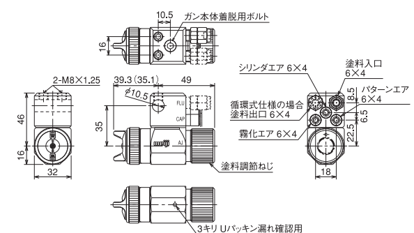
AJ 操作回路はp.10のE
