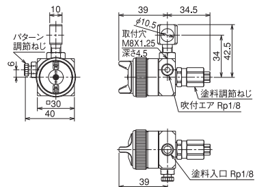
SA110 操作回路はp.10のC
