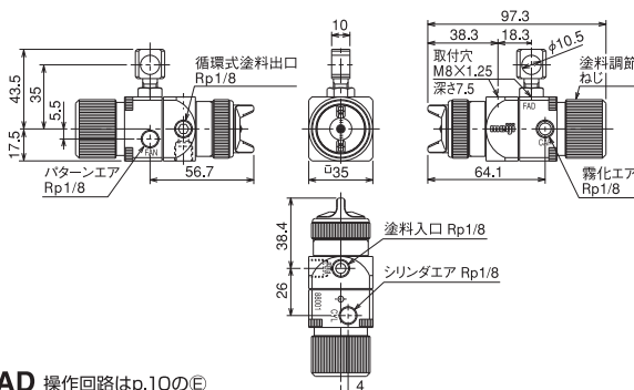
FAD 操作回路はp.10のE
