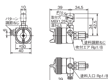
SA110 操作回路はp.12のC
