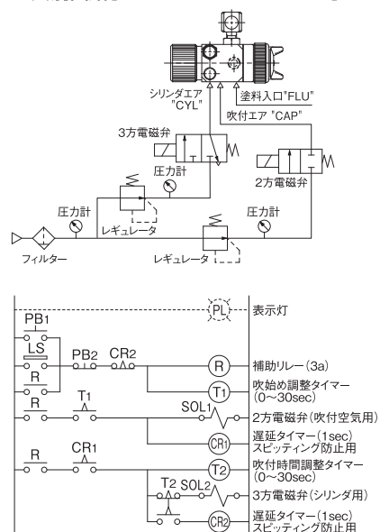
⑧シリンダ空気別回路[A110・A210・A110L・A55]
