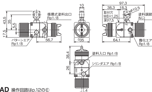
FAD 操作回路はp.12のE
