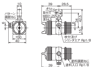
JA110 操作回路はp.12のC
