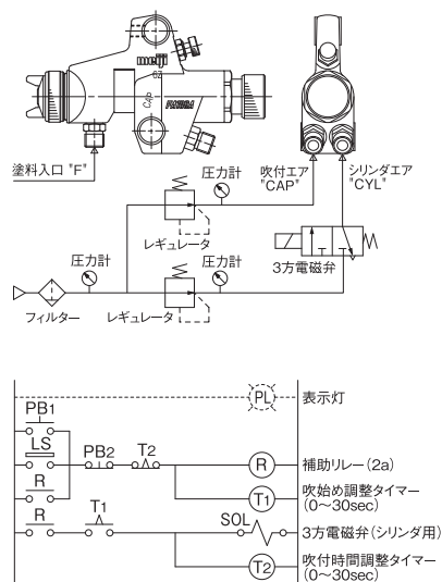
④吹付空気弁内蔵[FA110・FA210・FA110L]
