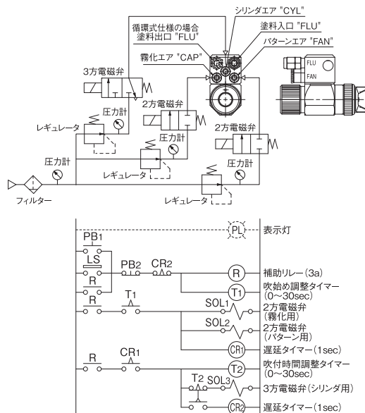
⑦ シリンダ空気別回路+パターン別回路[AJ]
