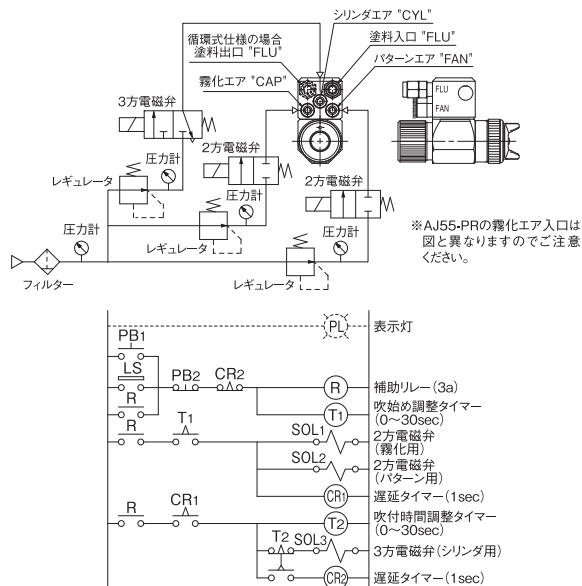
⑥ シリンダ空気別回路+パターン別回路 [AJ・AJ55]
