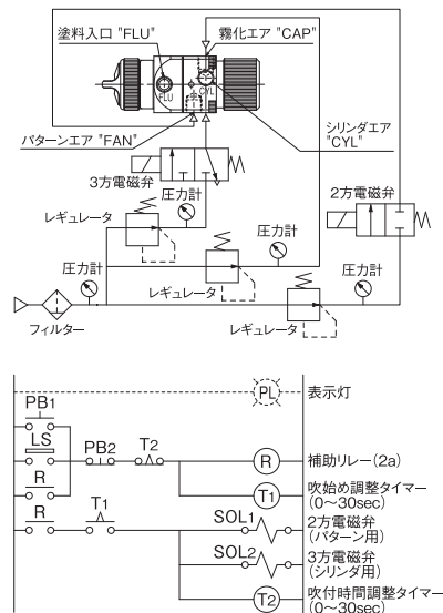
⑤ 霧化エア用空気弁内蔵+パターン別回路 [FAD]
