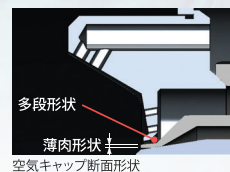
多段階形状 薄片形状 空気キャップ断面形状
