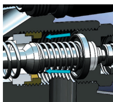
塗料溜まり防止構造 交換性を高めた「カートリッジ式ニードルパッキン」
