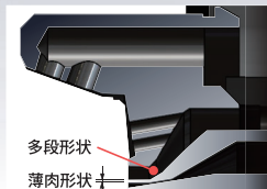
多段階形状 薄肉形状 FINER-CORE-HVLPタイプの 空気キャップ断面形状
