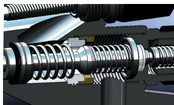
塗料溜まり防止構造 交換性を高めた「カートリッジ式ニードルパッキン」
