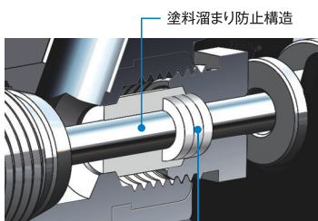
塗料溜まり防止構造 交換性を高めた「カートリッジ式ニードルパッキン」
