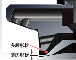
空気キャップ断面形状
