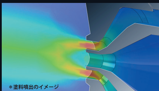
新型ノズル 多段整流機構を備えた先端薄肉ノズル形状
