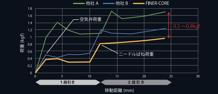
引金荷重曲線 (ガン入り口圧 0.2MPa) 他社ガンと比較した引金荷重の軽減 (約 30%軽減)
