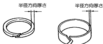
ピストンリングの厚さ測定
